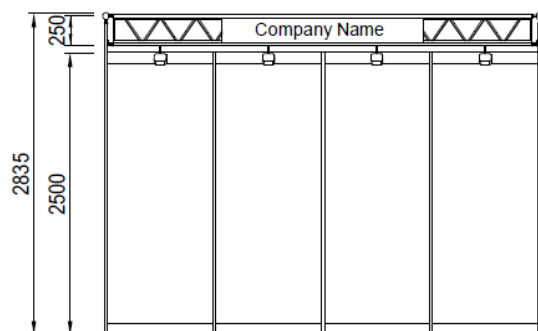
Ansicht
