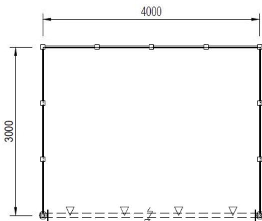
Grundriss (Beispiel: 4m x 3m)
